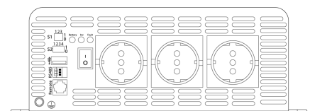
OUTPUT side
